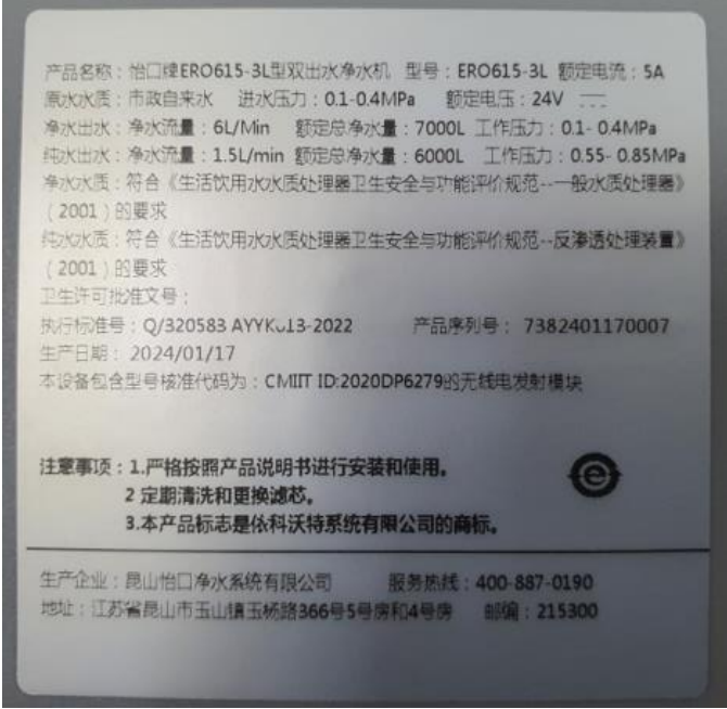
ER0615-3L (铭牌)
